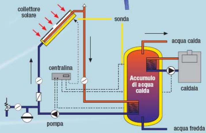
Schema di collegamento per funzione riscaldamento con integrazione caldaia
